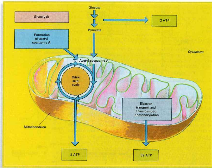
(شكل ١) الميتاكوندريا: المصنع الذي يقوم بتكسير الاسيتايل كوانزيم - أحد أنواع نواتج الجلوكوز - في دورة كريس ثم يحولها إلى السلسلة التنفسية أو سلسلة نقل الالكترونات لإنتاج مادة الأدينوسيك ثلاثي الفوسفات
