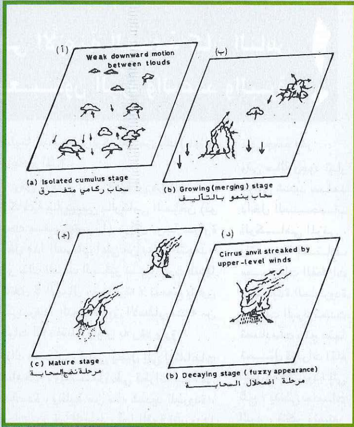
شكل (٤) : رسم توضيحي يبين مراحل تكون السحاب الركامي المزمي
