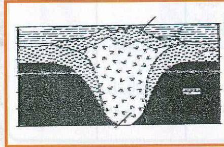
شكل (٢) يوضح جذراً بازلتيا من قشرة محيطية منغرس في طبقة الوشاح .
