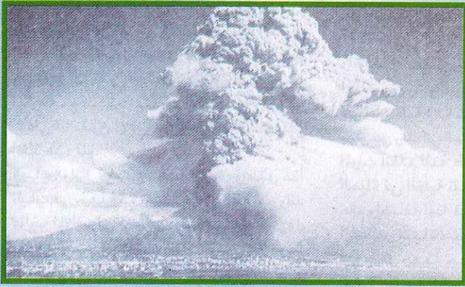
شكل (١) : صورة تبين السحاب الركامى المزنى ويلاحظ أنه يشبه الجبل فى تكوينه ، تبين الصورة أيضا ارتفاع مباني المدينة مقارنة بارتفاع السحاب
